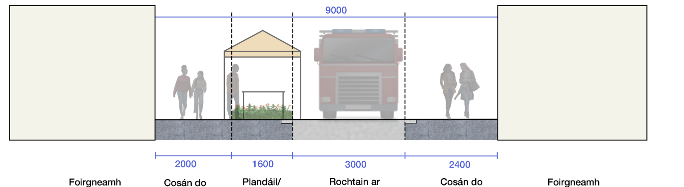
Rannóg Margaídh/Ócáide na Sráide Trasna (FF')
