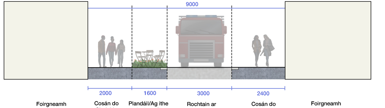
Rannóg na Sráide Trasna (EE')
