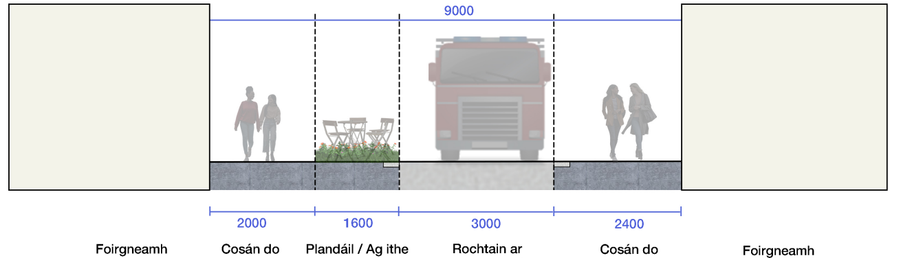
Rannóg na Sráide Trasna (DD')
