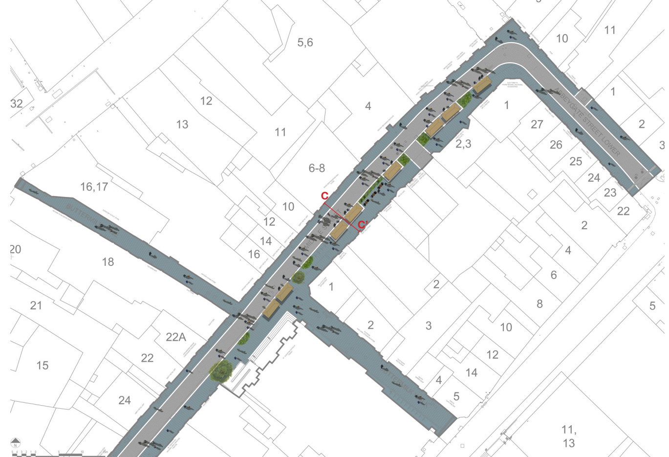
Rannóg Margaídh/Ócáide na Sráide Láir (CC')
